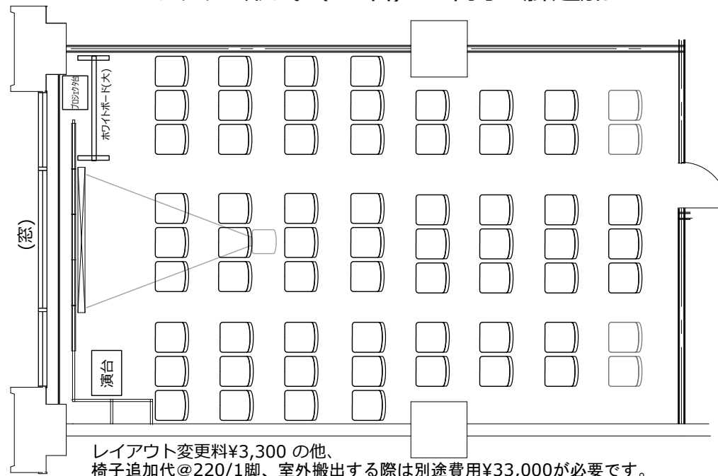
シアター形式 (64名) ※椅子4脚追加
